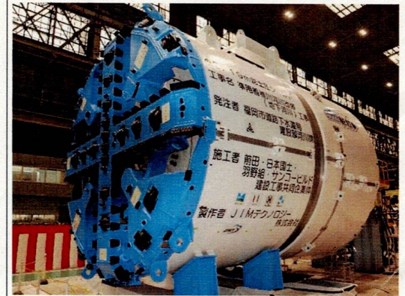
シールドマシン（工場制作時）
